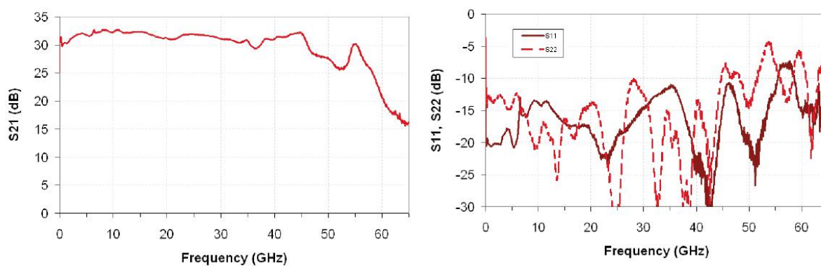
图 2 S 参数
