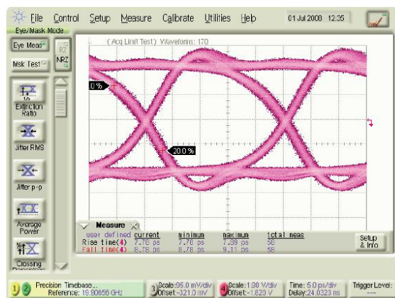
图 1 40Gbps 眼图
