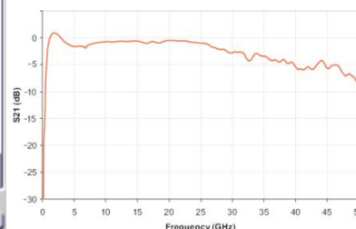
图 3 S21 曲线
