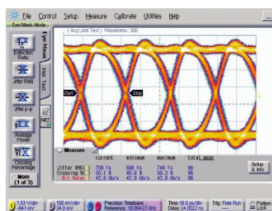
图 2 40Gbps 眼图
