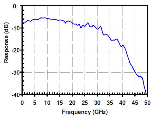
图 2 S21 曲线
