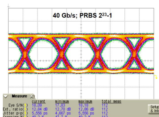
图 1 40Gbps 眼图
