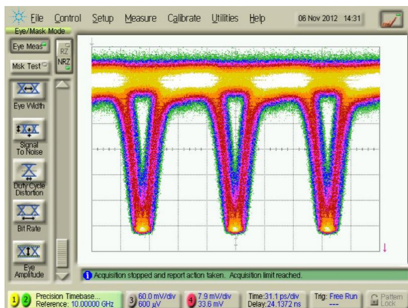
图 1 10Gbps 眼图
